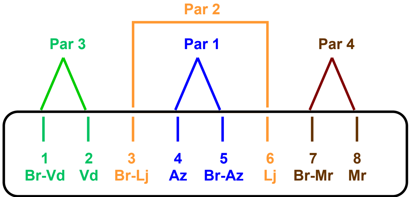
T568A
