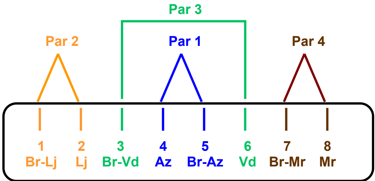
T568B
